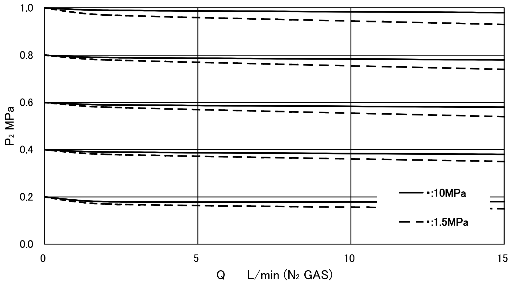
S-LABO-0,S1,B1sr P 2 -Q (0.6MPa,1MPa,1.5MPa計) 特性
